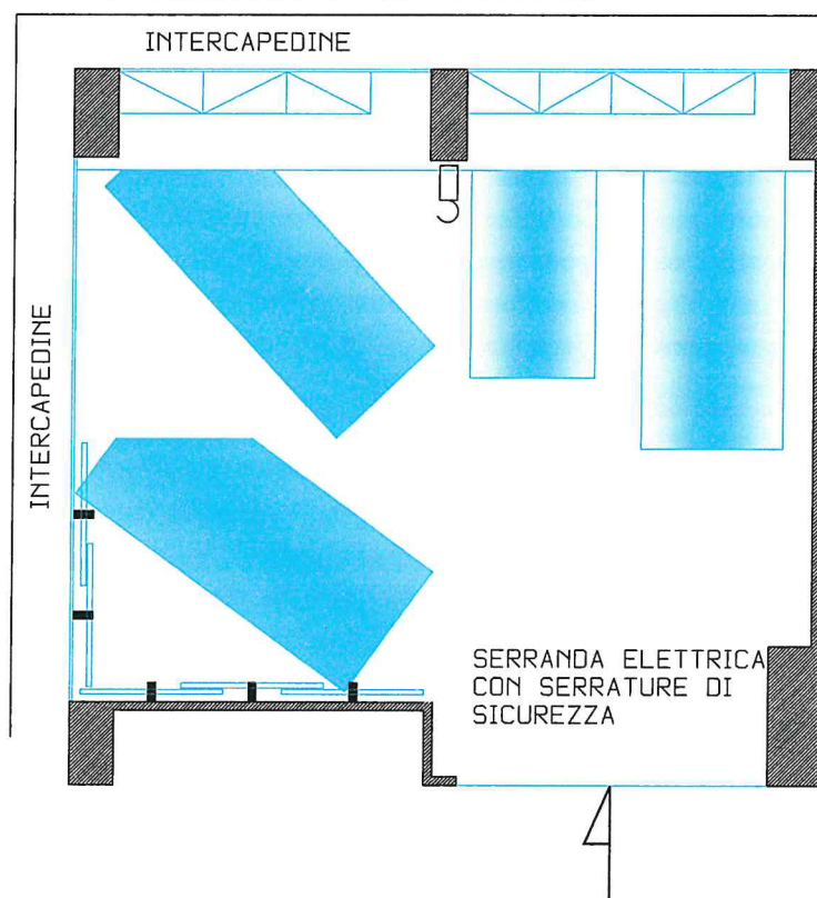
SOPPALCO CON SCAFFALI IN METALLO E ARGANO ELETTRICO MQ.7,60; TENDONI A SCORRIMENTO ANTIPOLVERE
